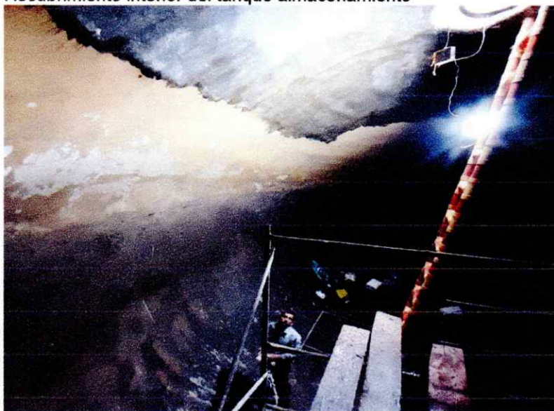
Recubrimiento interior del tanque almacenamiento
